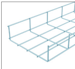
DZ - výška 50, \emptyset drátu 4 mm, rastr pole 50 x 100 mm
