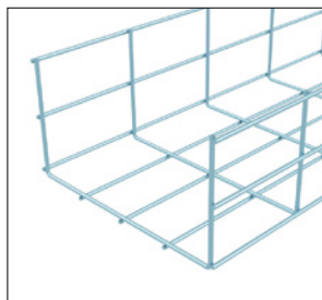
DZ - výška 100, \emptyset drátu 4 mm, rastr pole 50 x 100 mm
