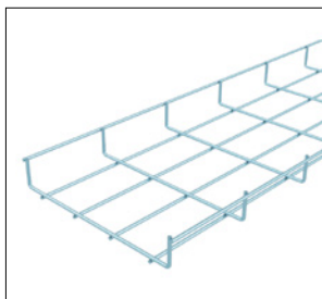
DZ - výška 30, \emptyset drátu 4 mm, rastr pole 50 x 100 mm
